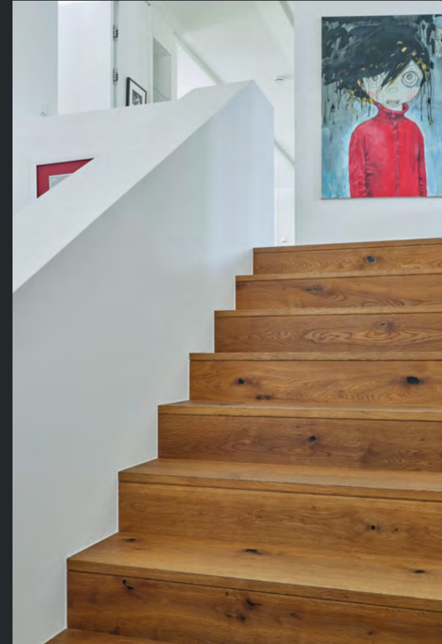
Tritt- und Setzstufe mit Schattenfuge
